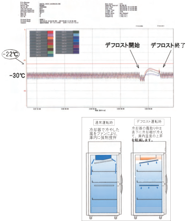
温度分布：設定温度（常用温度-30℃）
