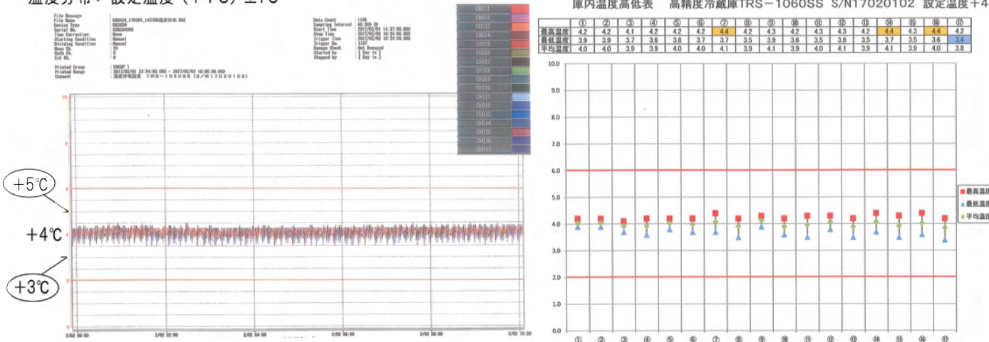
温度分布：設定温度（+4℃）±1℃
