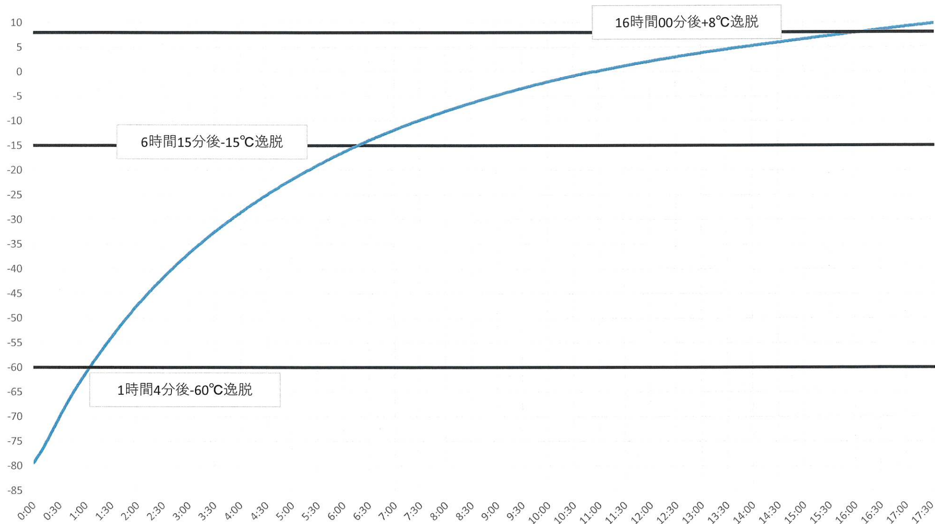
UD-80W74NF 無負荷時庫内温度推移(外気温+23°C)
