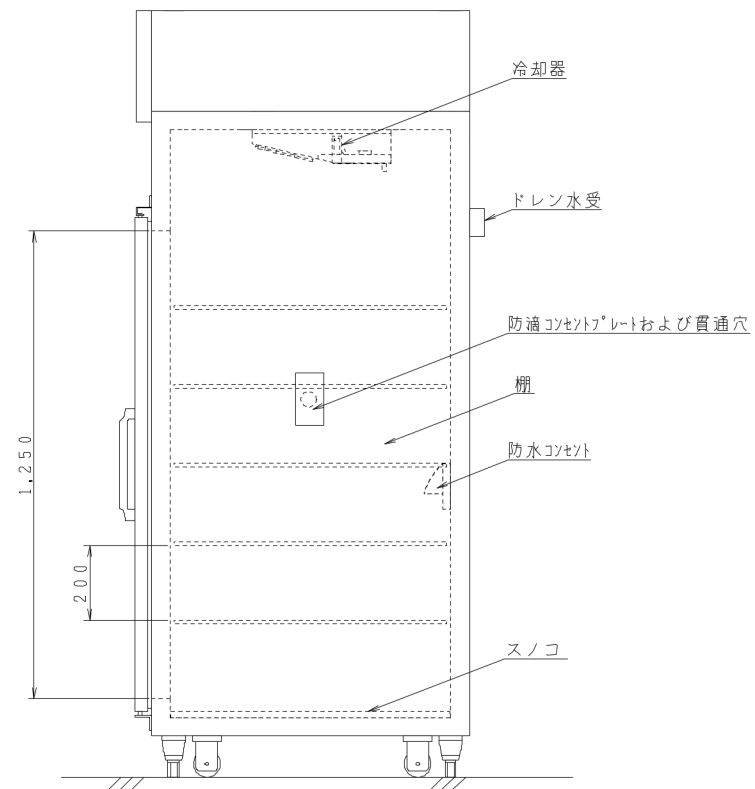
側面図
