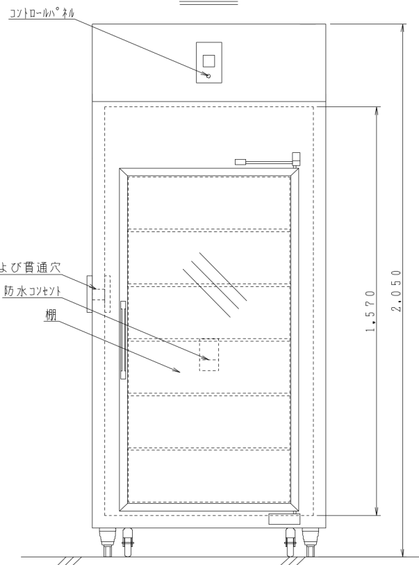
正面図
